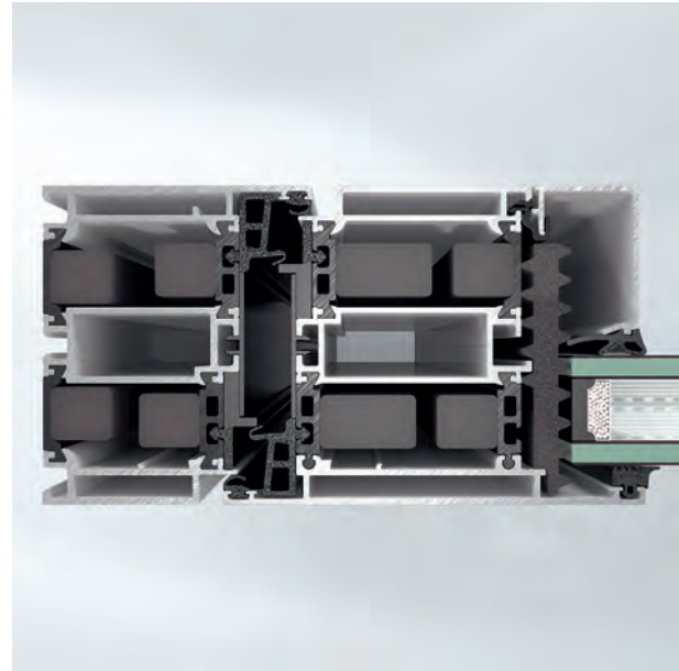
Schüco Door ADS 90.SI SimplySmart
