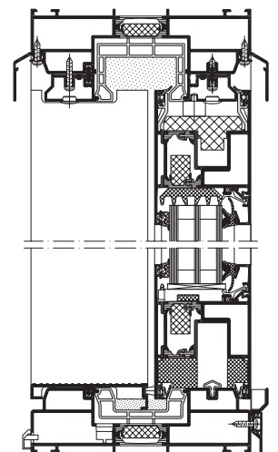
Schüco ASS 70.HI, scale 1:5
