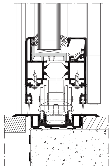
Schüco ASS 70 FD, scale 1:2
