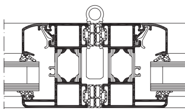
Schüco ASS 70 FD, scale 1:3
