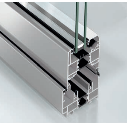
Schüco ASS 70 FD
